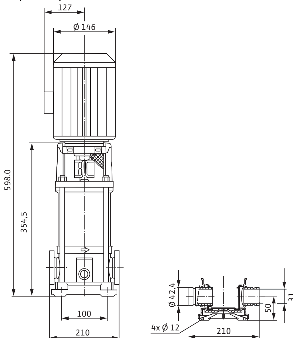
Габаритный чертеж
